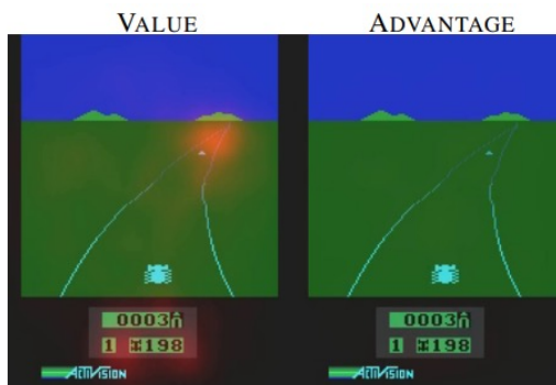
状态价值函数 Advantage函数
